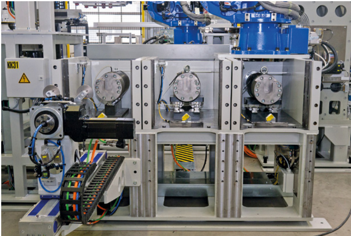
In den Werkzeugaufnahmen sichern drei Schreibleseköpfe den Einsatz der korrekten Werkzeuge
